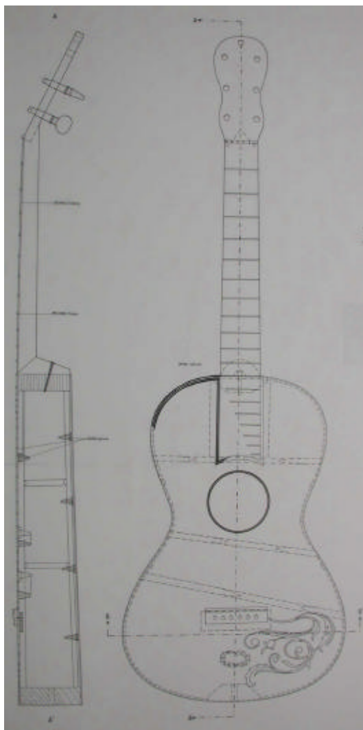
Detalj av teknisk tegning for Schöne-gitaren
